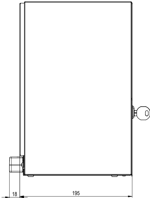
Zijaanzicht
